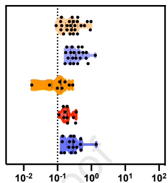
SARS-CoV-2-N
