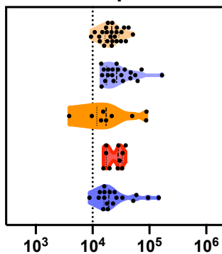
RSV-preF
